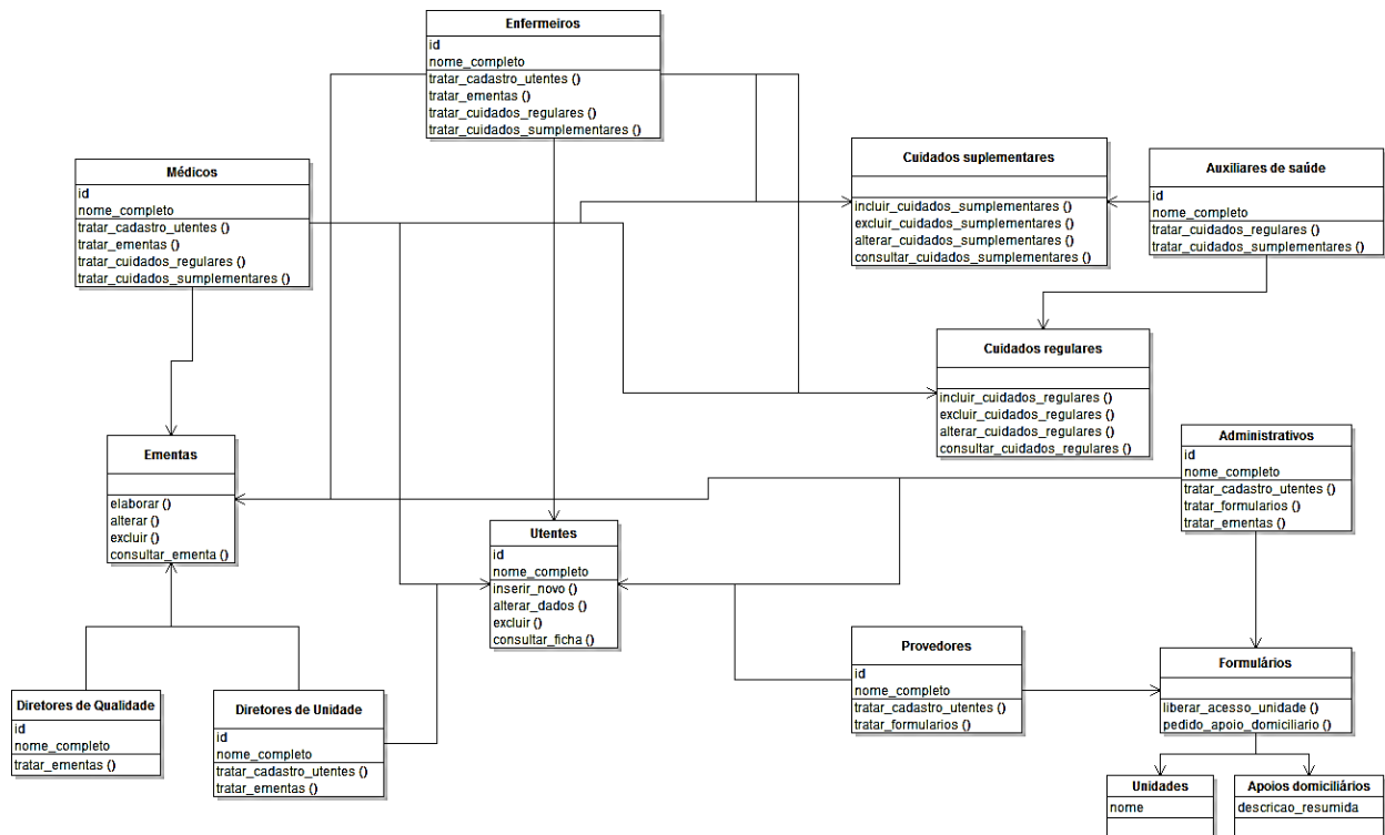
Figura 39 - Diagrama de Classes inicial para "2. Gerir Utentes"
