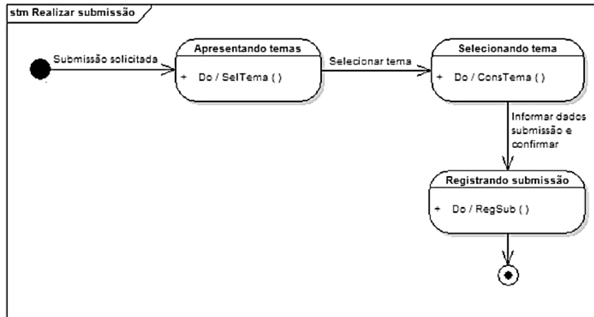
Figura 8 - Diagrama de Estados Guedes [2005, p.11]
