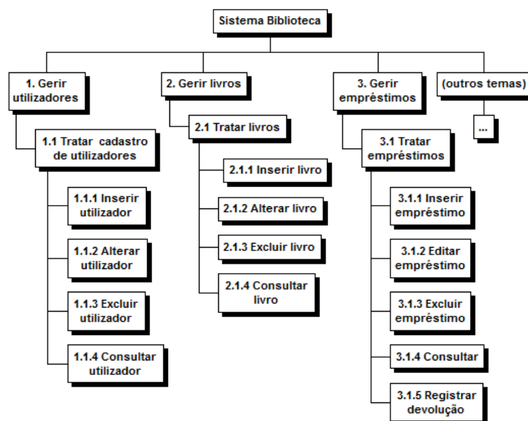
Figura 29 - Exemplo de trecho de WBS para um Sistema de Gestão de Biblioteca
