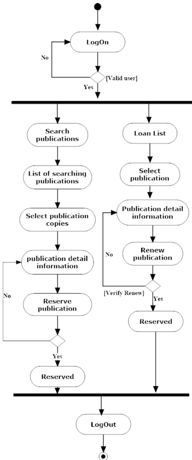
Figura B.29 - Activity Diagram (Renovar e Reservar Publicações)
