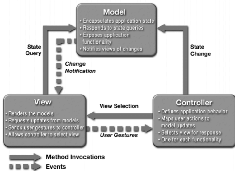
Figura 2.21 - Padrão MVC [53]
